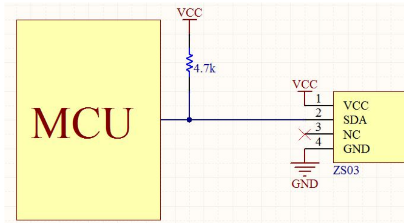
图 3: 应用电路
