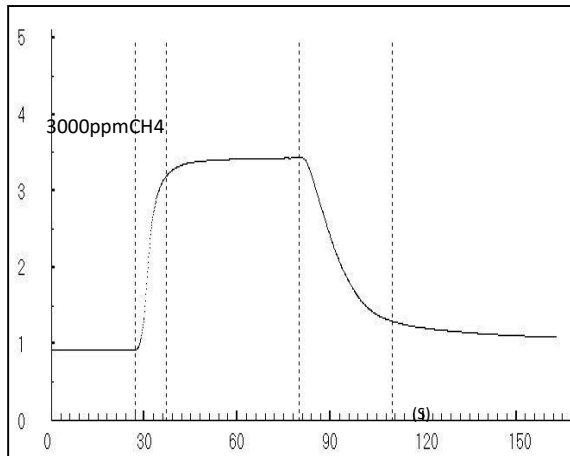
图5：响应恢复曲线图
