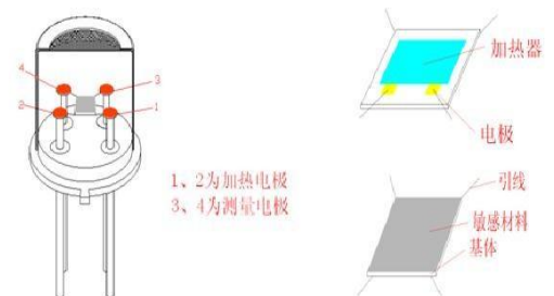
1: 传感器结构图
