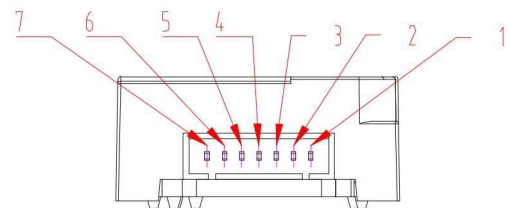
图 4 管脚定义
